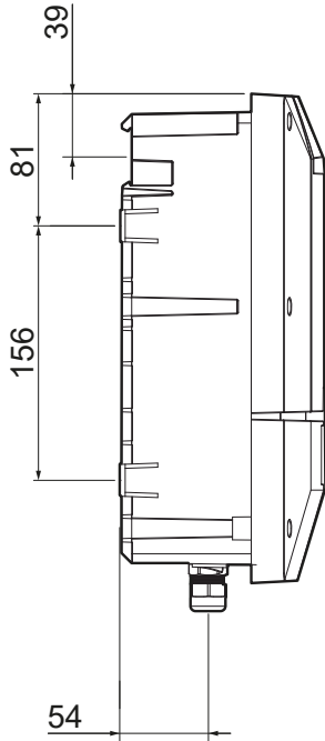
Zijaanzicht
