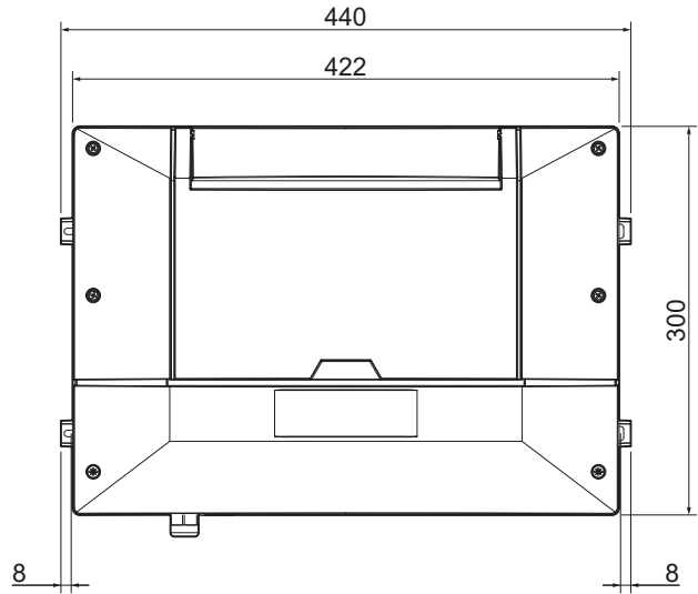
Vooraanzicht
